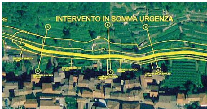
L'area di Mori dove verrà realizzato il vallo-tomo a protezione delle case
